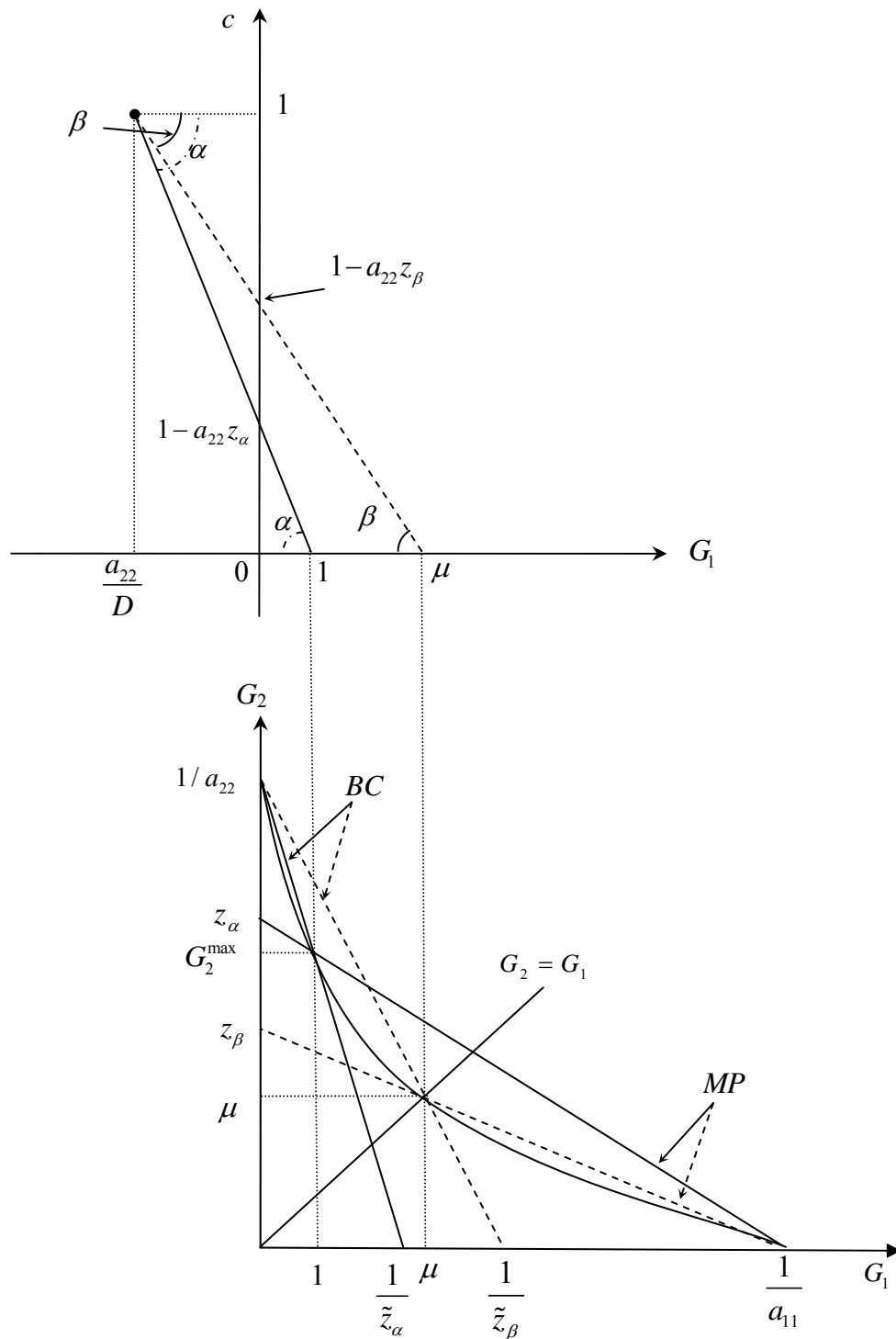
Figure 2 : Le cas où le déterminant D est négatif
