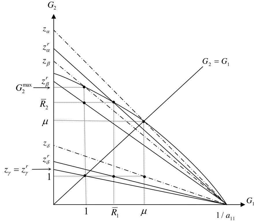
Figure 5 : Les proportions critiques de Marx
